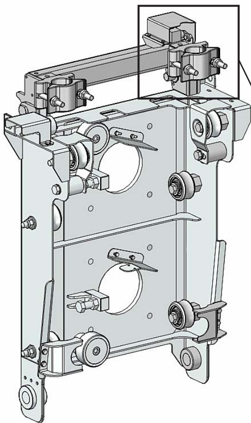
Рисунок 6.3.7 Защитные зажимы прикреплены к мачтовым трубам на время проведения работ под кабиной.
