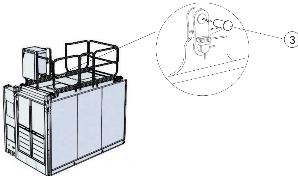
Рисунок 6.3.2 Снятие защитной крышки (А) и крепежных штифтов (Б).
