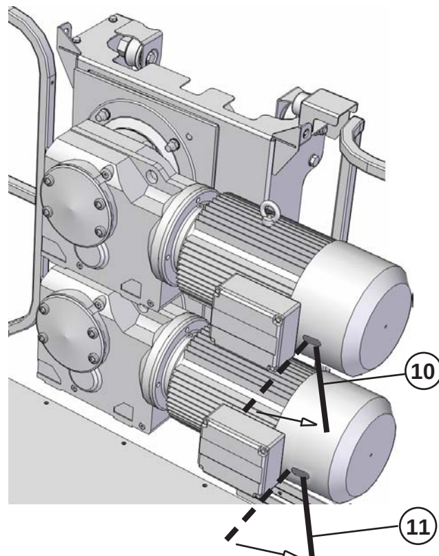
Рисунок 6.3.5 Опускание подъемного механизма
