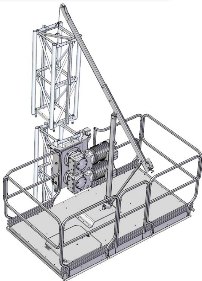
Рисунок 6.4.1 Монтаж мачты
