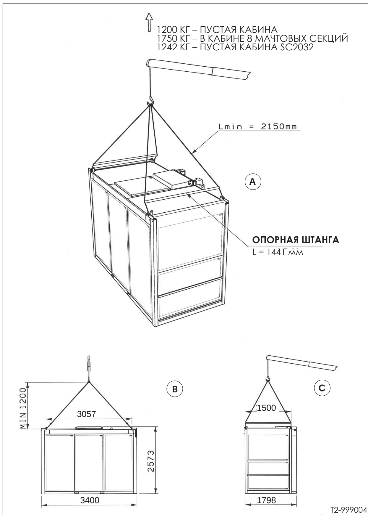
Рисунок 6.1.1 Поднятие кабины подъемника с петель
