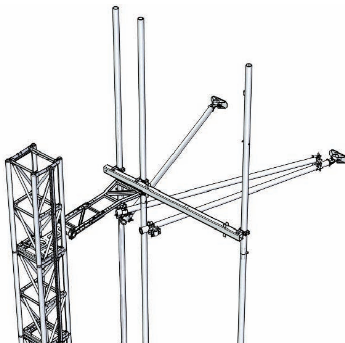
Рисунок 6.5.2 Линия труб
