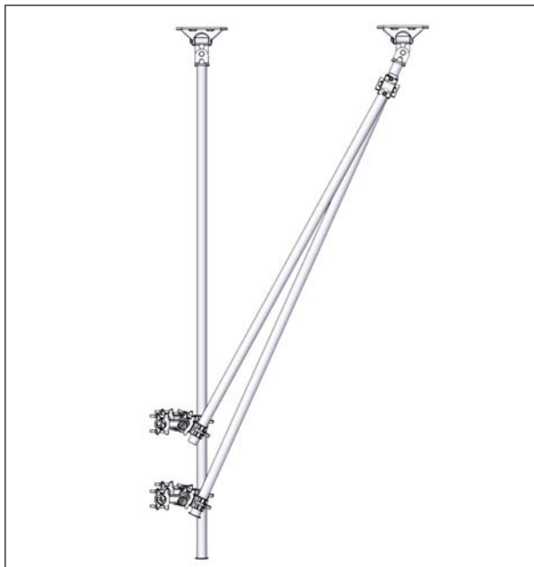
Рисунок 6.2.2 б) PG124639 Верхний анкер
