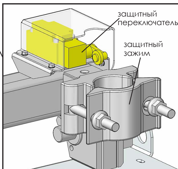
Рисунок 6.3.7 Защитные зажимы прикреплены к мачтовым трубам на время проведения работ под кабиной.
