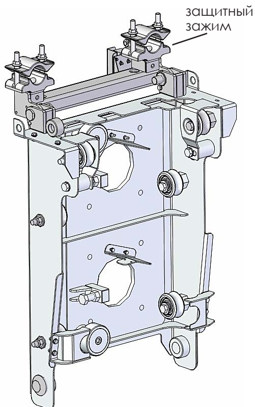
Рисунок 6.3.6 Положение защитных зажимов, когда подъемник работает.
